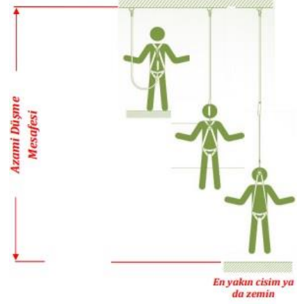
Emniyet kemeri, bağlama tertibatı ve enerji emici
